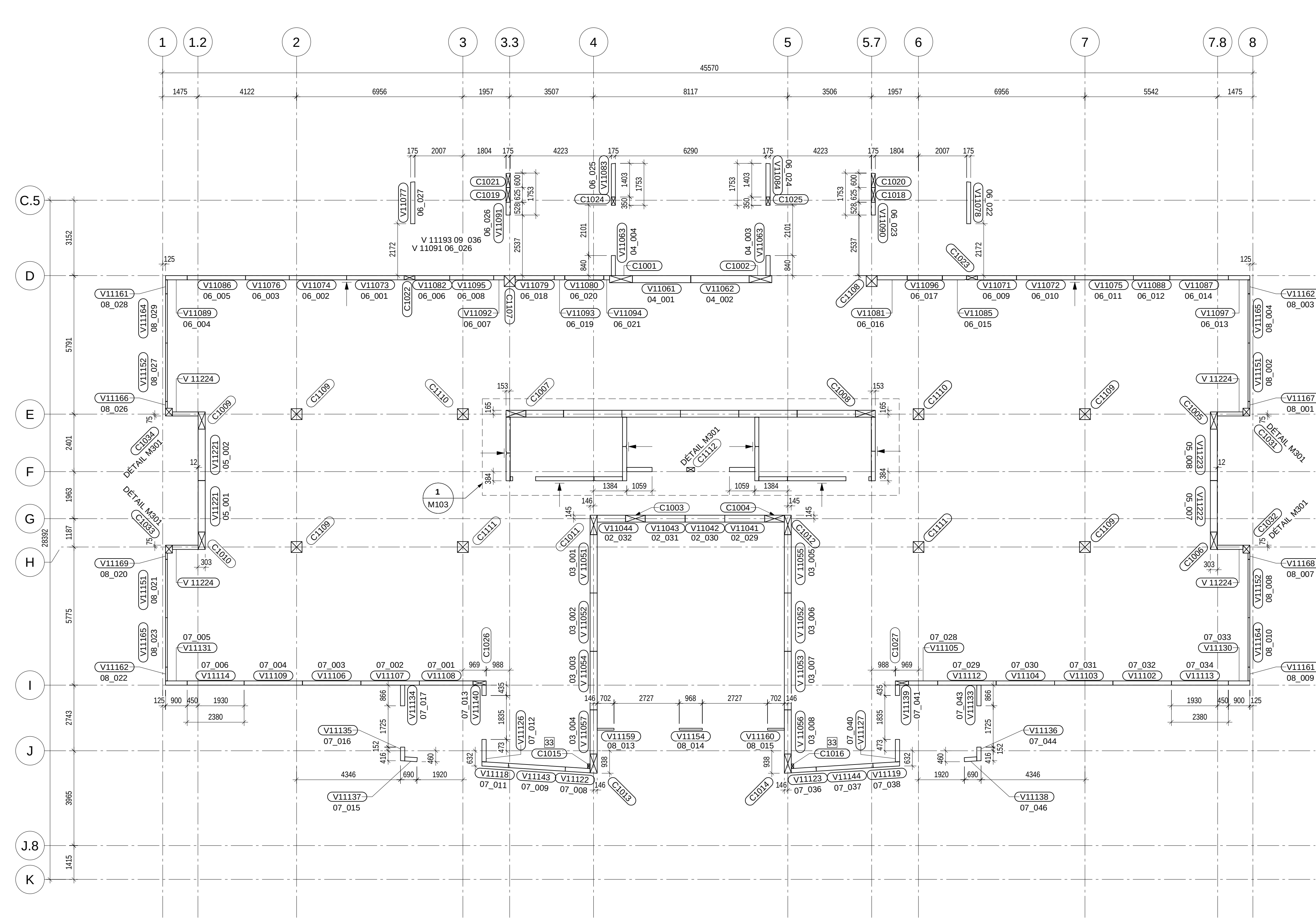
PLAN DE COLONNES ET MURS NIVEAU 1 ÉCH.: 1: 100
